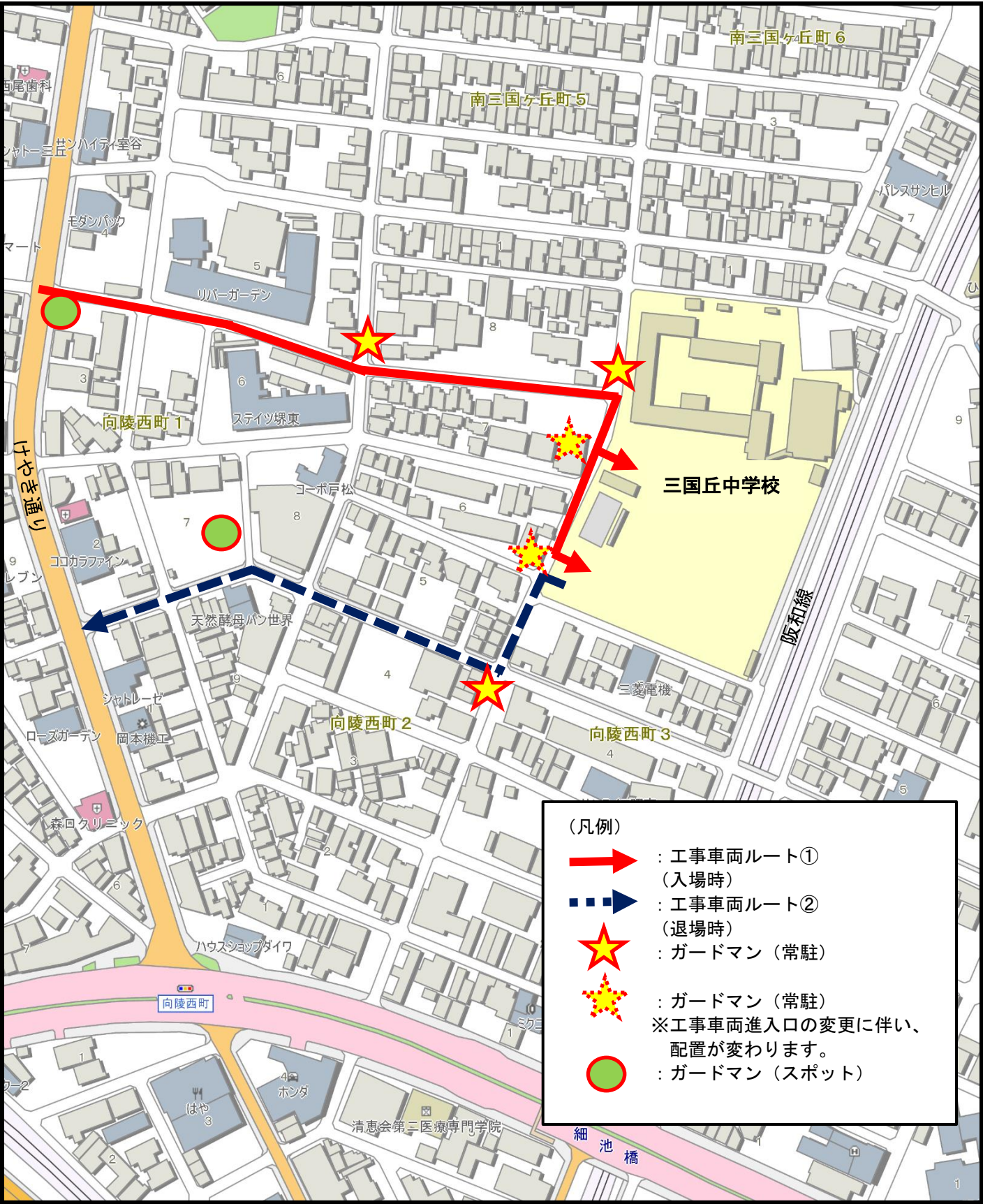
＜改築工事時の工事車両ルートについてR7.10頃～（予定）＞
